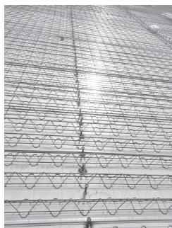
钢筋桁架楼承板
