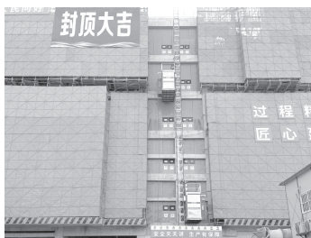
施工升降机楼层电梯门全网片封闭
